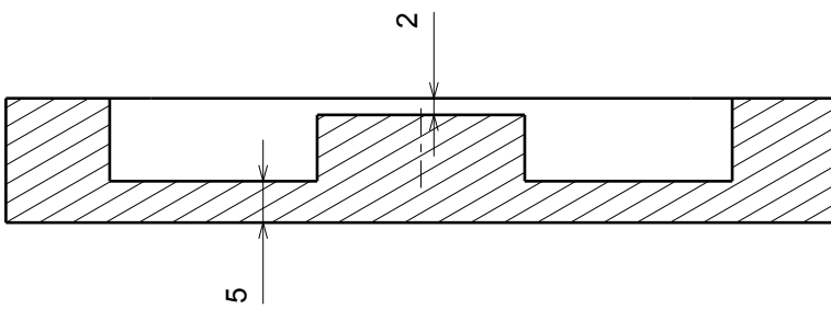
Section view A-A Scale: 1:1
